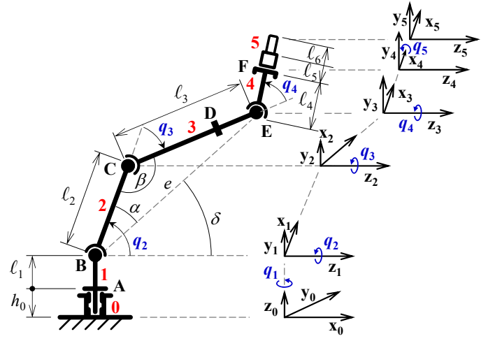
Fig. 4. Scheme of the DH coordinate frames.
